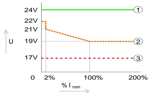
Afbeelding 4-2: Dynamisch DC-ingangsvenster
