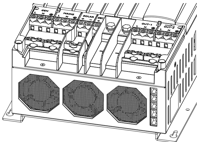
Afbeelding 5-3: Deksel verwijderd
